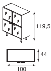
Шкаф без топа, черное стекло 117 8040 1897
