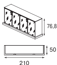
Низкая стеклянная шкафовая композиция без топа 151 5050 2119
